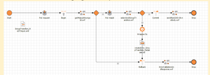
BPMN Prozess mit Verzweigung, und Subprozesse.
